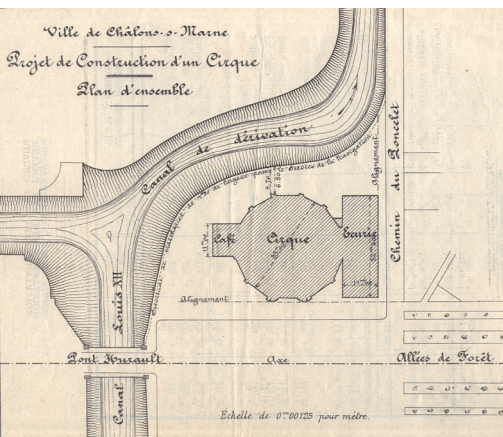
Projet de construction du cirque de Châlons par Louis Gillet. © Archives Départementales de la Marne, fonds Gillet 84 J 5.
